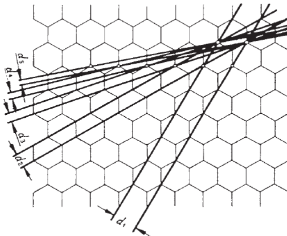
Fig. 6. Espaciamento interplanar en grafito.
